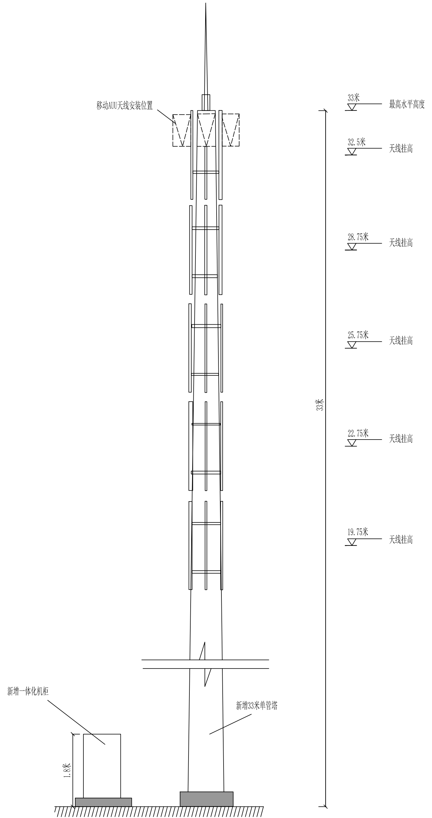
基站正视图
