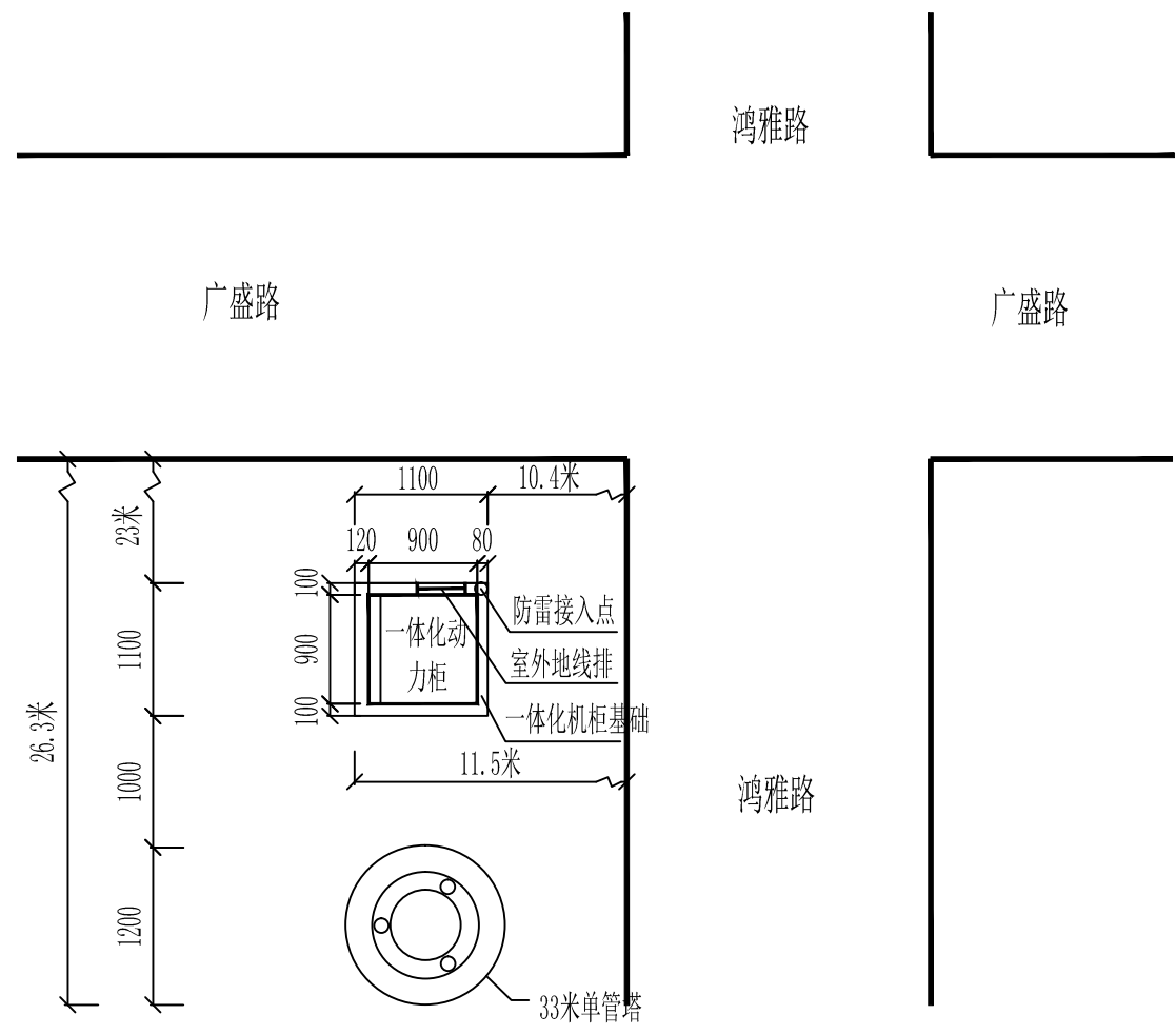
平面图
