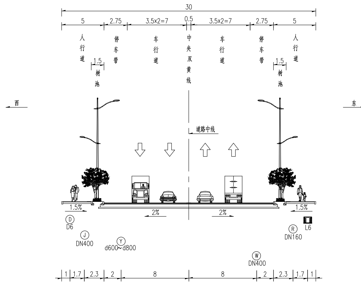
鸿雅路管线综合标准横断面图 (推荐方案)
