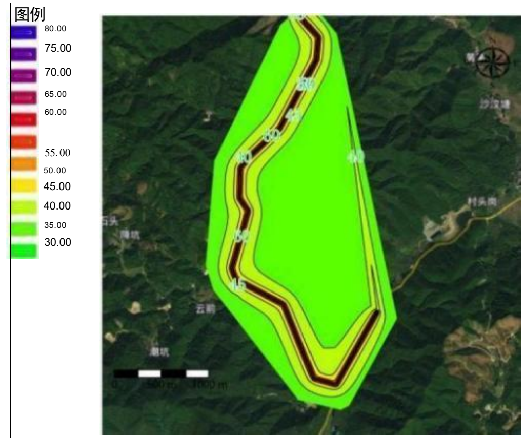
图5.2-2-4项目等声值线图(2030年夜间噪声贡献值, 未采取隔声降噪措施)
