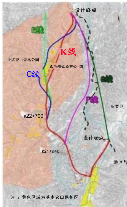
图2-3各路线比选方案平面图
