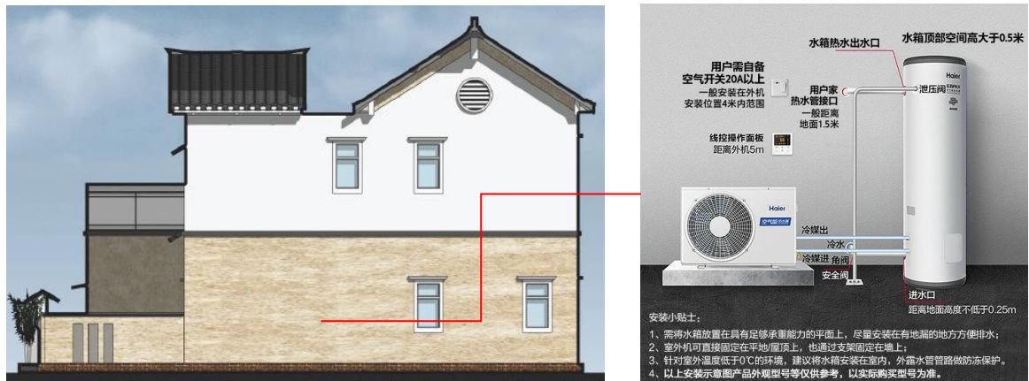
图A.0.4-5 绿色农房空气源热泵示意图
