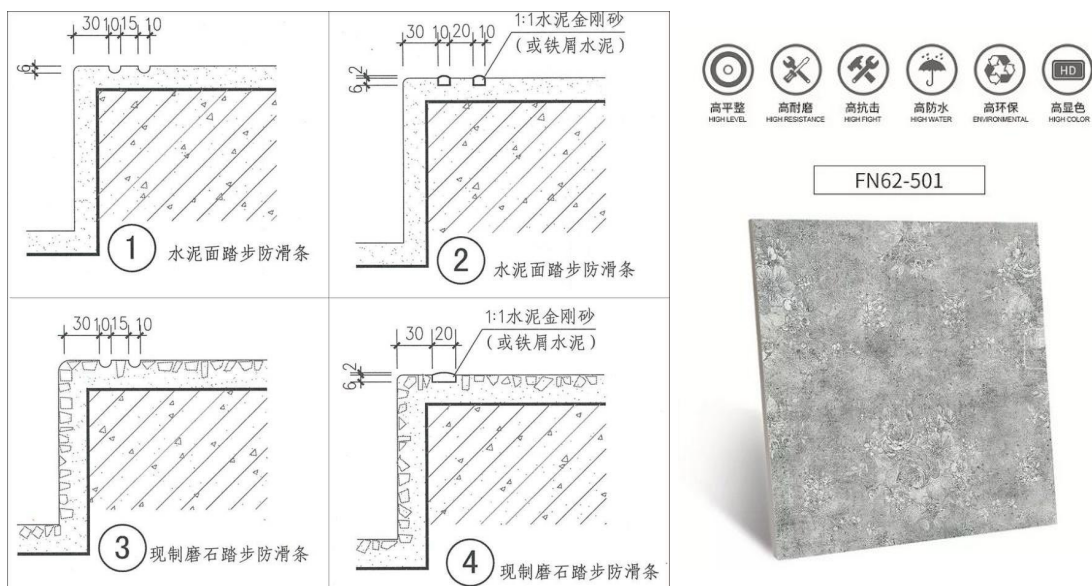
图 A.0.1-4 踏步防滑示例
