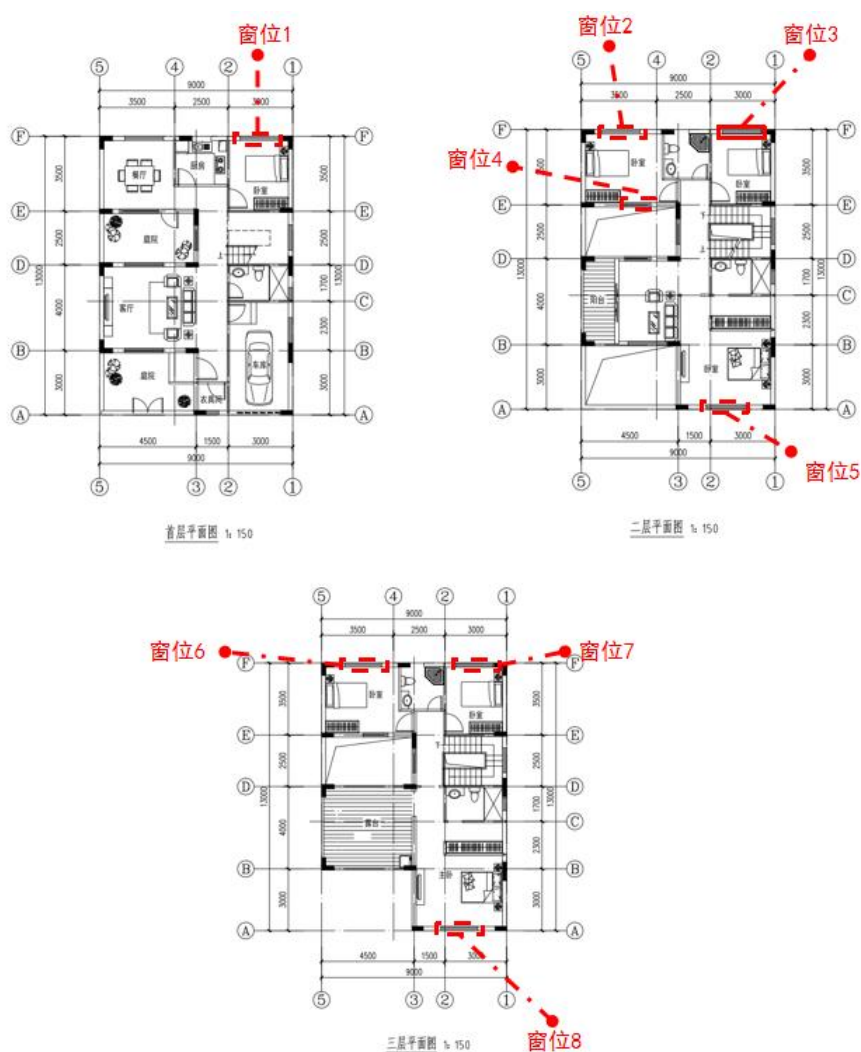
图A.0.2-3 绿色农房窗位布置示例
