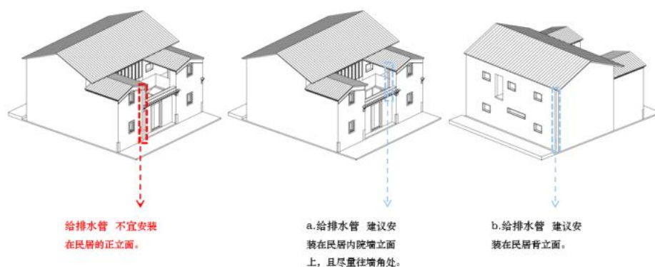
图A.0.2-2 绿色农房排水组织措施示例
