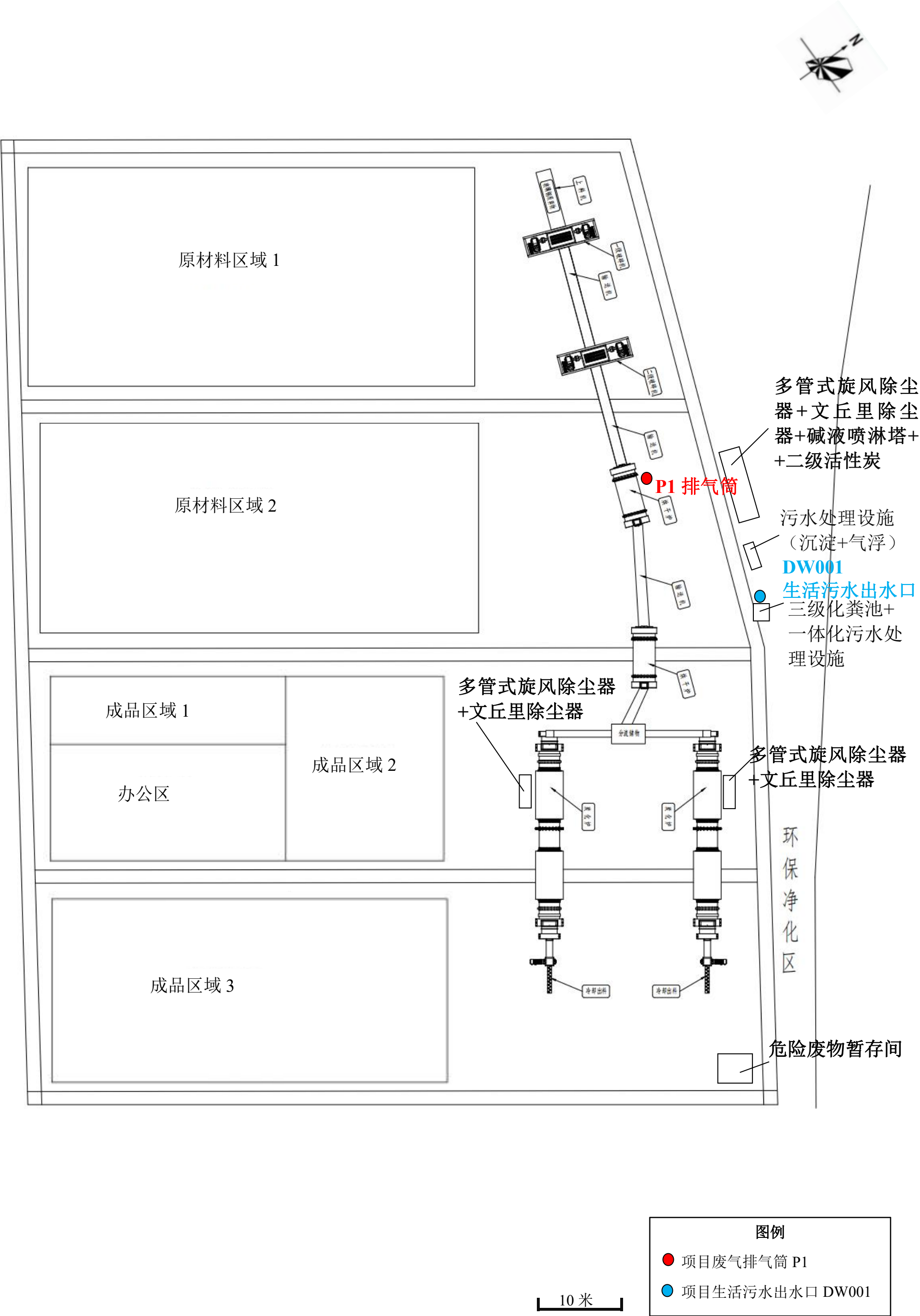
附图 3 项目平面布置图
