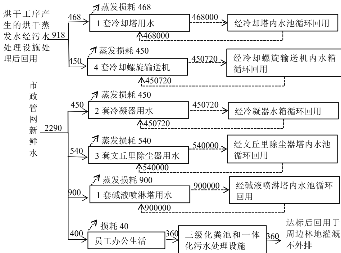
图 2-1 项目营运期水平衡图 （单位：m 3 /a）
